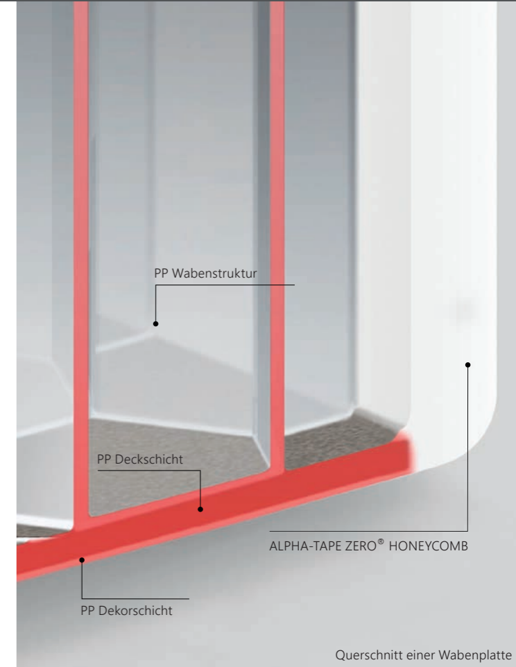
Querschnitt einer Wabenplatte
